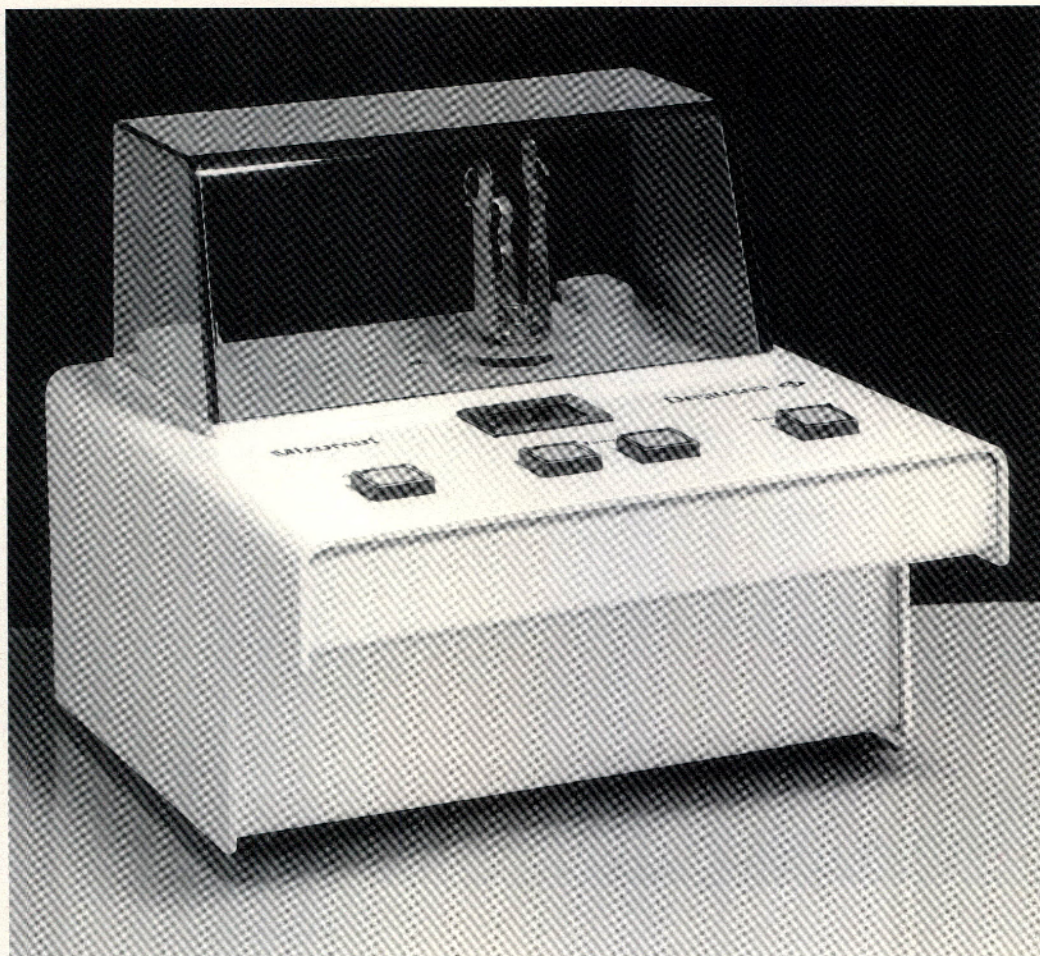
De Mixomat van Degussa is een mengtoestel voor alle typen capsules en spuiten met amalgaam en andere vulmaterialen. De elliptische mengbeweging zorgt voor een optimale menging.
